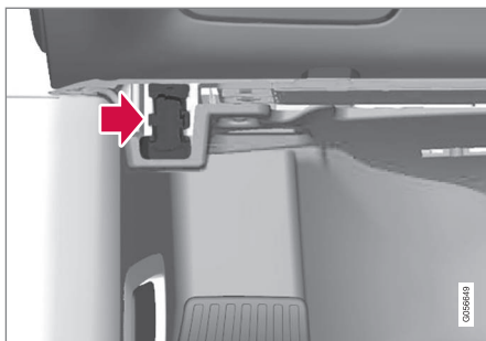
La toma de diagnóstico está situada debajo del tablero de instrumentos en el mismo lado que el volante.
